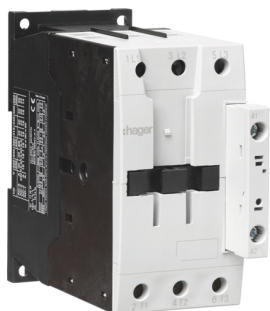
EVXX_SIZE3_3P
